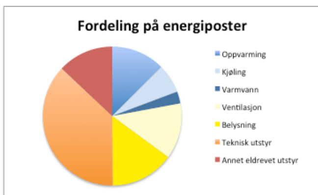
Figur. Eksempel på energibudsjett for beregnet reelt energibehov (dvs bruk av reelle verdier og ikke standardverdier) for et passivhus/ A-merket kontorbygg på 107 kWh/m 2 år. Oppvarming utgjør 13,5 kWh/2, som for dette bygget dekkes med varmeoverskudd fra byggets datasentral. I praksis er kjøpt energi i dette bygget 95% elektrisitet og sparepotensialet ligger i å redusere dette. (Kilde: Grønn Byggallianse)
