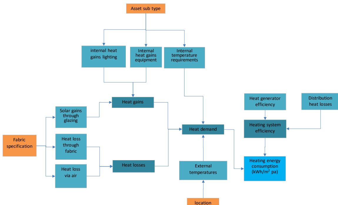
Figur 3: Skjematisk fremstilling av forenklet energimodelleringsstilnærming for romoppvarming
