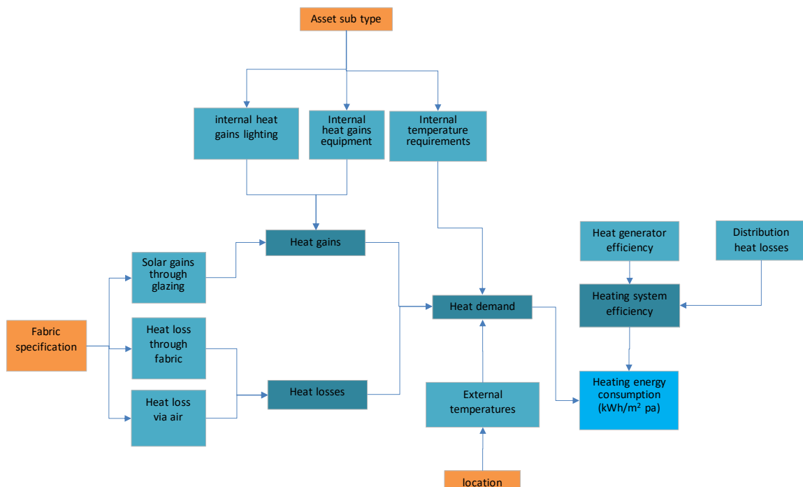
Figur 3: Skjematisk fremstilling av forenklet energimodelleringsstilnærming for romoppvarming
