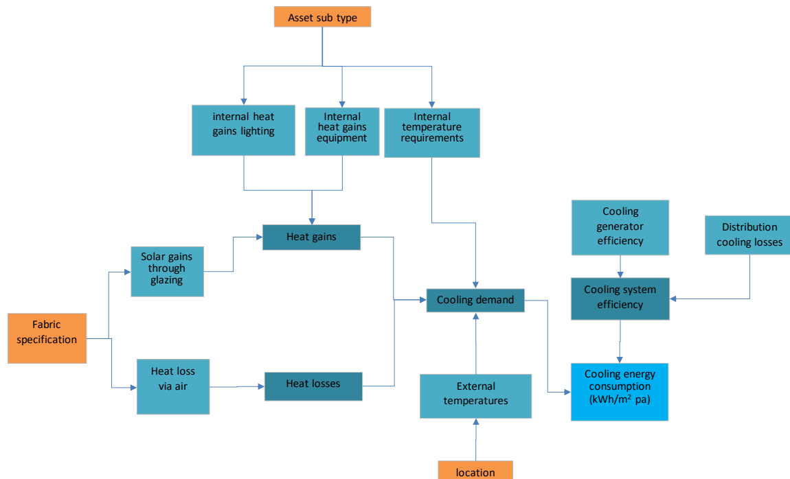
Figur 4: Skjematisk fremstilling av forenklet energimodelleringsstilnæring for kjøling
