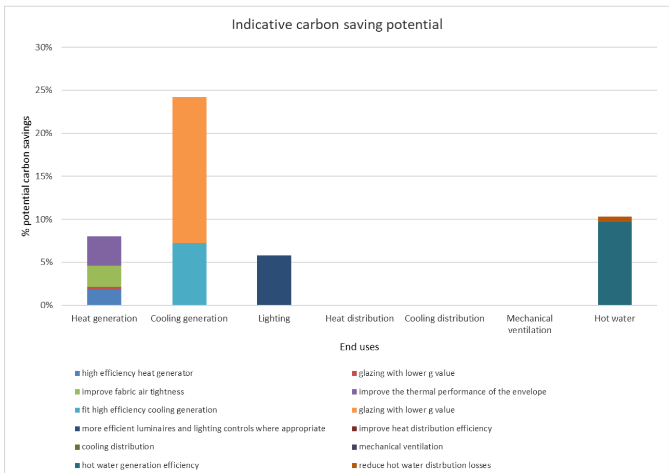
Figur 5: Eksempel på resultat – indikativt potensial for CO 2 -sparing
